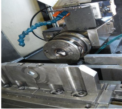
Beg gängrollmaskin Toolman-Conrit konstruktion, med utbytbara gängrollhuvuden Max gängdim M16
