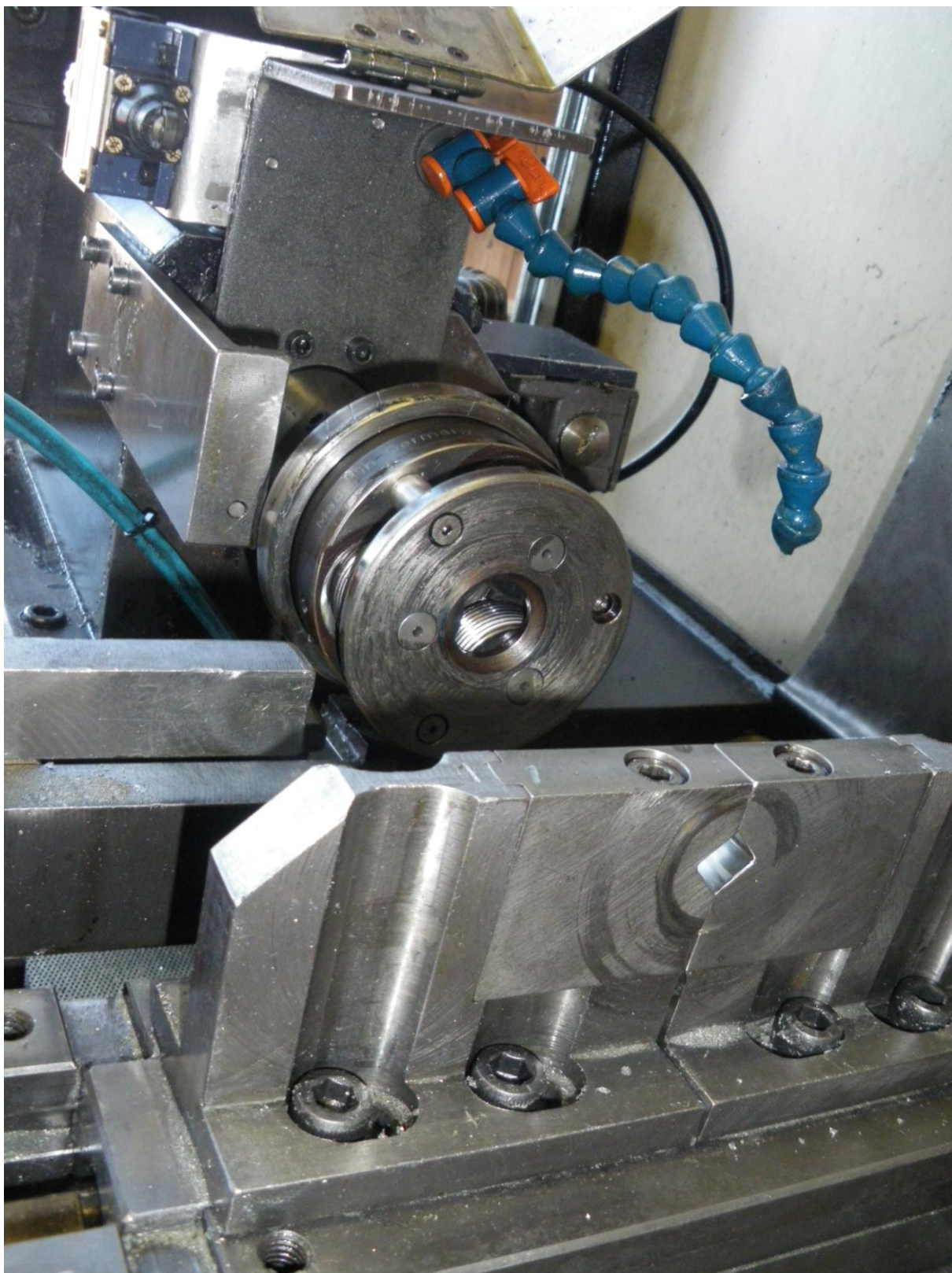
Beg gångrullmaskin Toolman-Conrit konstruktion med utbytbara gångrullhuvuden . Max gångrull M16
